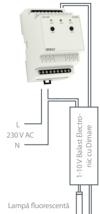
LBC3-02M Dimmer 1-10V pentru lămpi fluorescente
